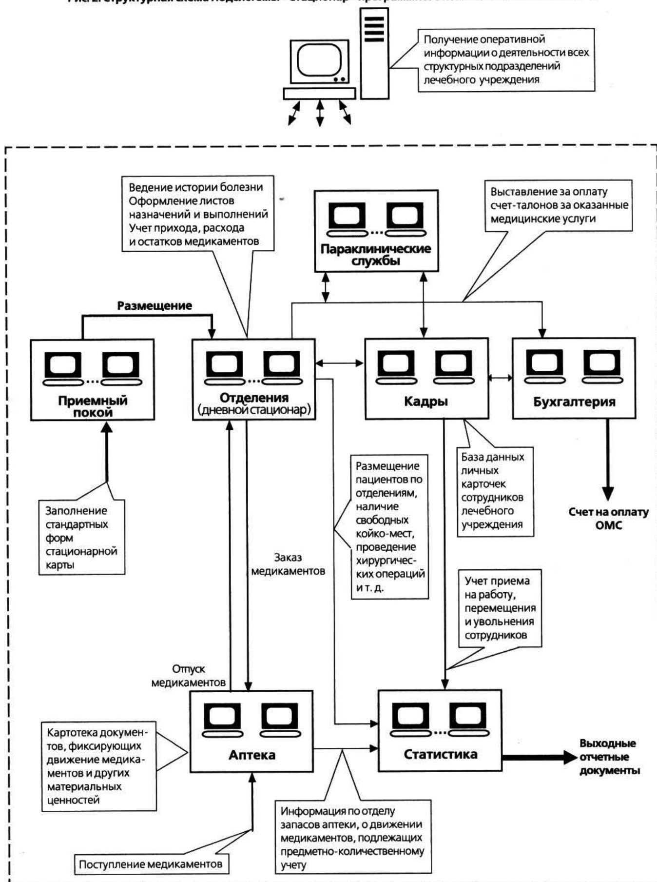
Рис. 2. Структурная схема Подсистемы «Стационар» программного комплекса «С-Госпиталь®».
